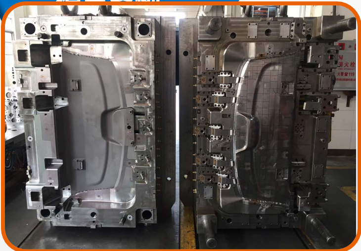
汽车零部件-行李厢衬里 Auto Part- Trunk Trim
