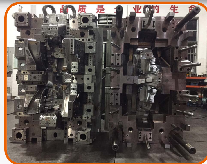
汽车零部件-车灯座 Auto Part-Lamp holder
