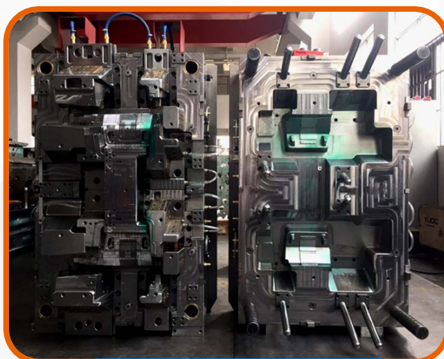
汽车零部件-内部零件 Auto Part-Internal Part
